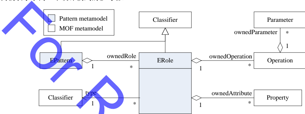
Fig.4 Pattern meta-metamodels
